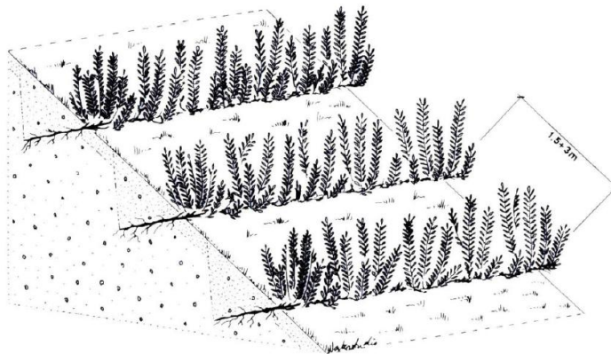
gradonata/cordonata viva - vista prospettica
