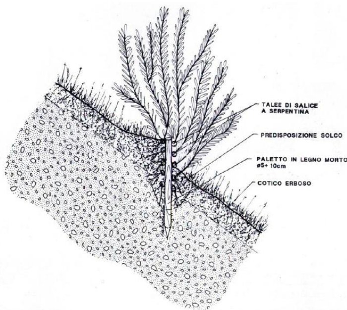
Viminata Viva - sezione tipo
