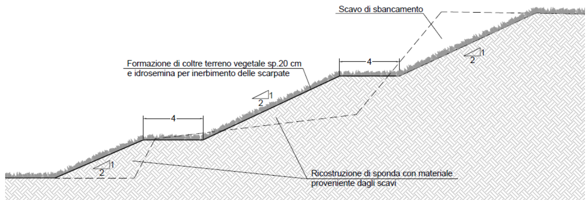
Esempio riprofilatura versante - Dettaglio tecnico a cura di Sogesid
