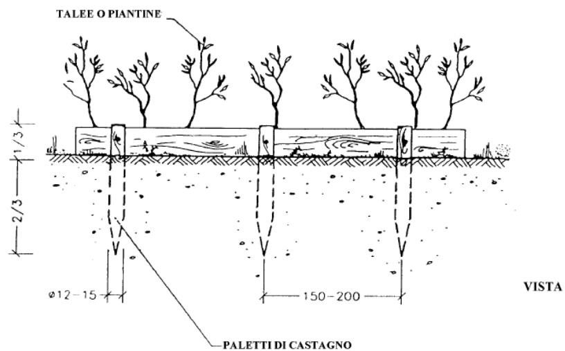
Palizzata viva - vista
