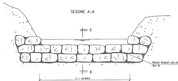
soglia in massi
