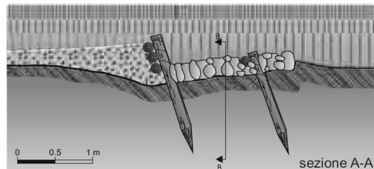
sistemazione a gradinata con soglie.
