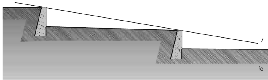
sistemazione a gradinata con soglie.
