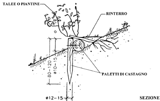
Palizzata viva - sezione
