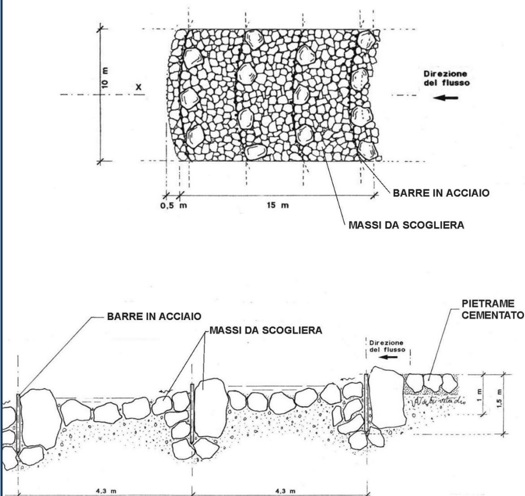
Rampa a blocchi (in pianta ed in sezione)
