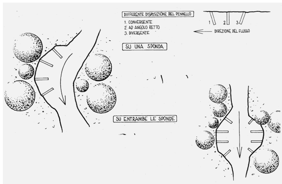
Pennelli (convergente, ad angolo retto, divergente)
