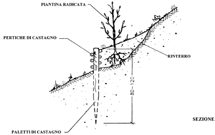
Graticcetta Viva - sezione tipo
