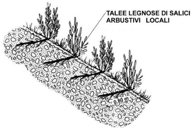
Massa a dimora di talee
